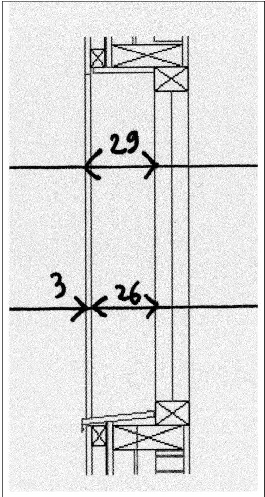
Coupe verticale sur menuiserie du RDC (extrait de la coupe AA)
