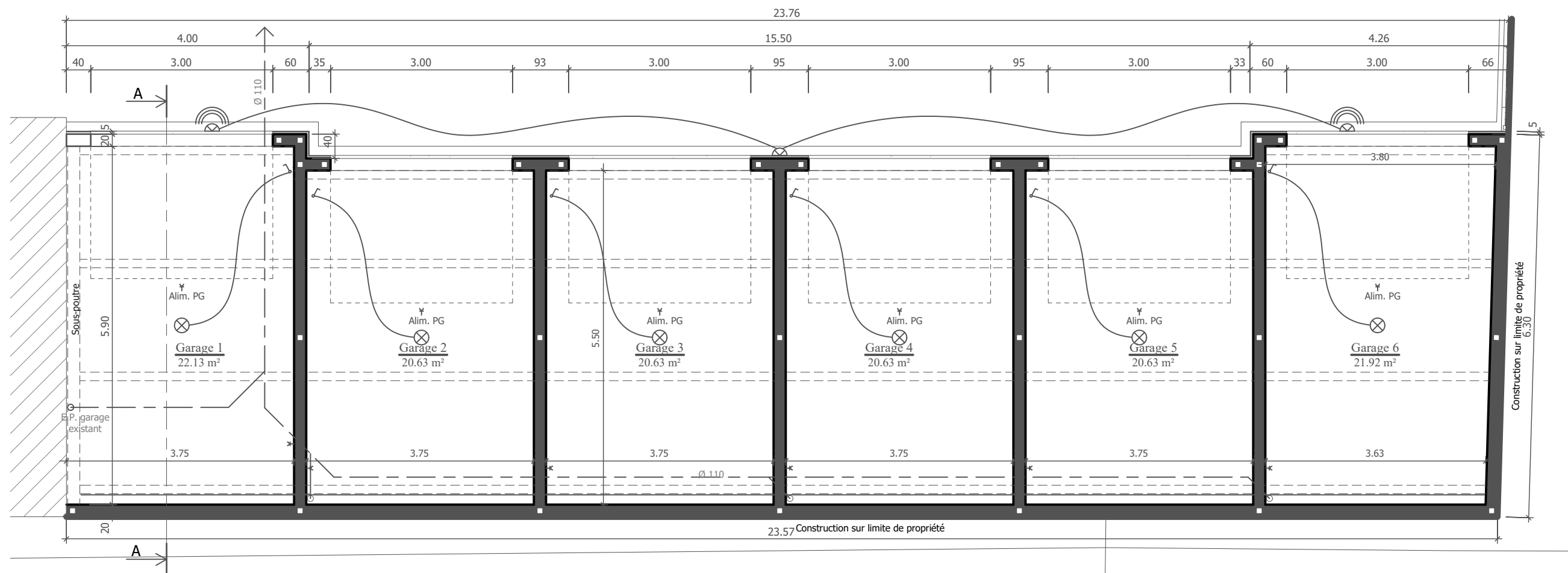
Vue en plan des garages en bande
