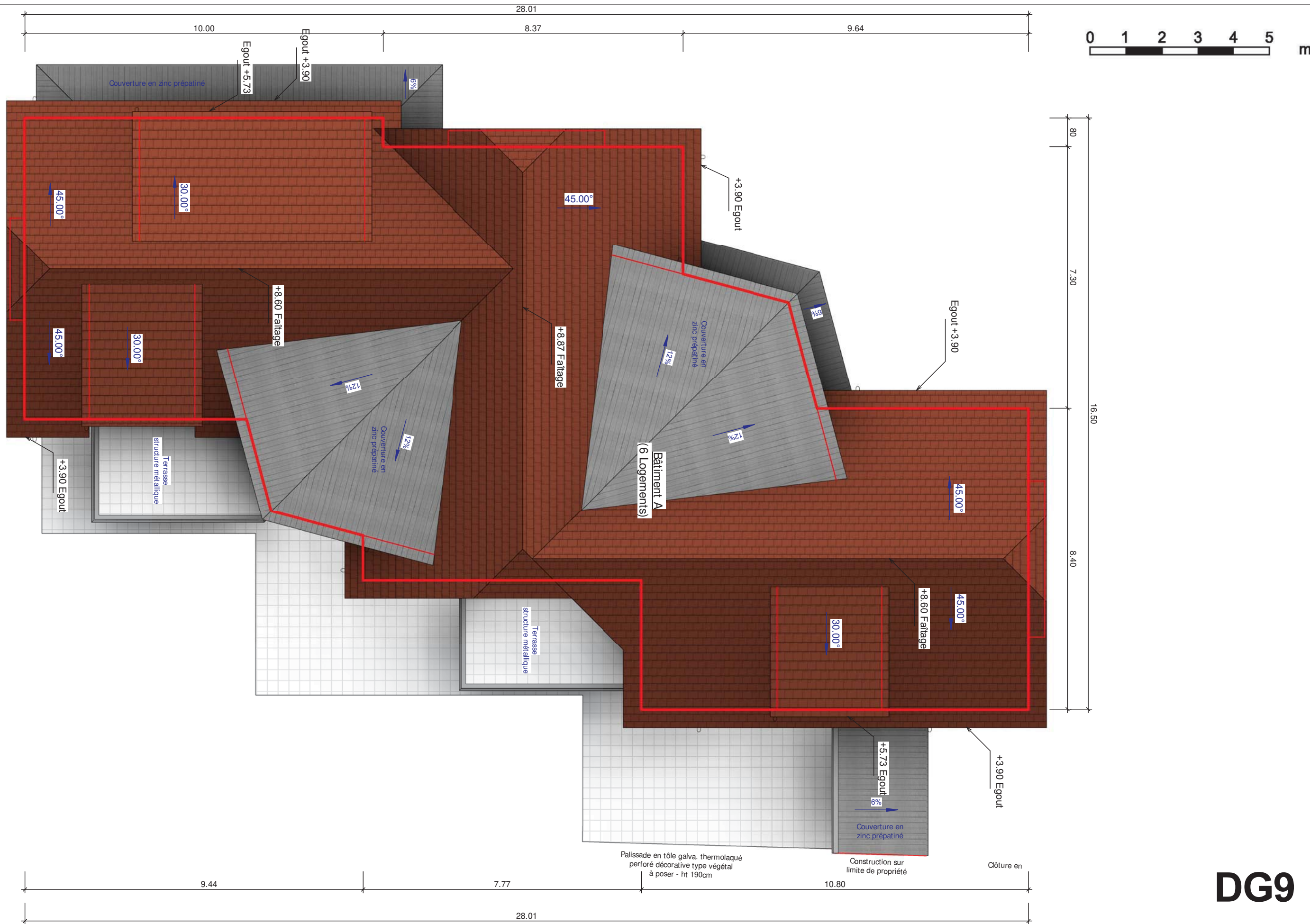
Plan de toiture - Bâtiment A
