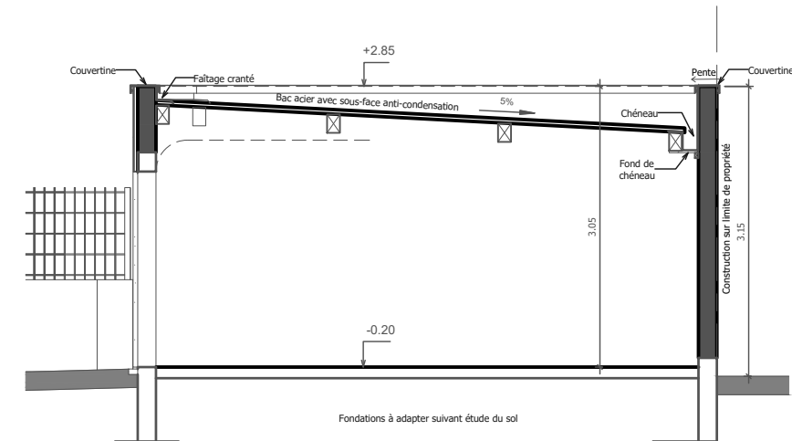
Coupe AA - Garages en bande
