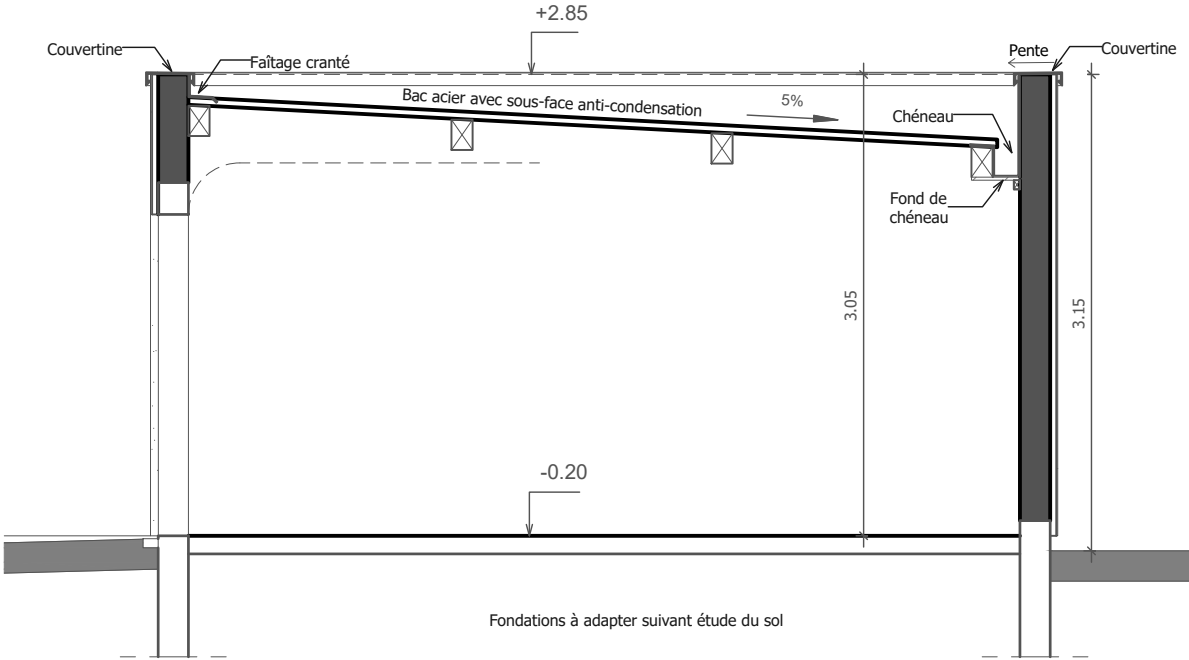
Coupe du garage individuel
